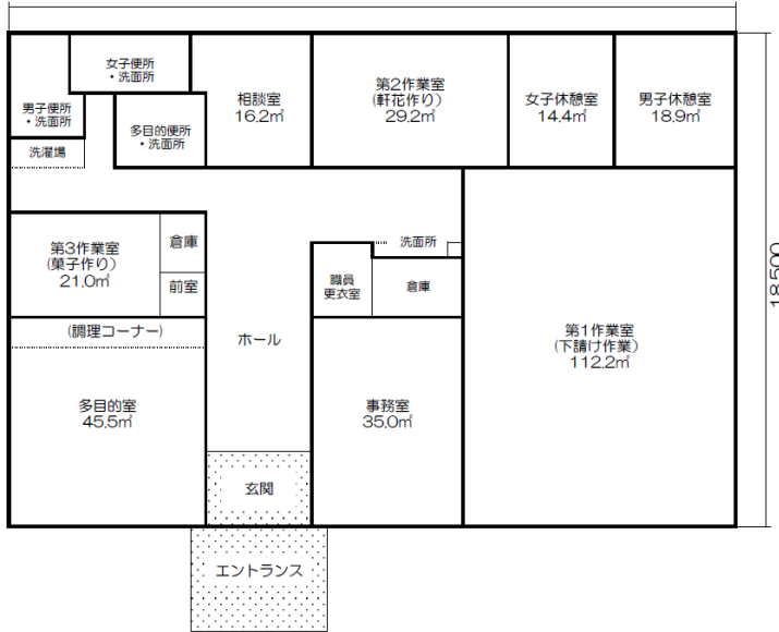
さから作業所平面図 23,800
